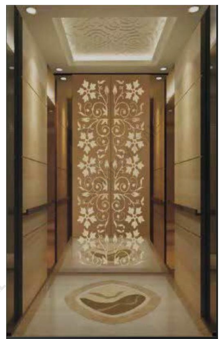
HD112
