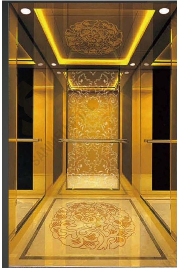
HD202
