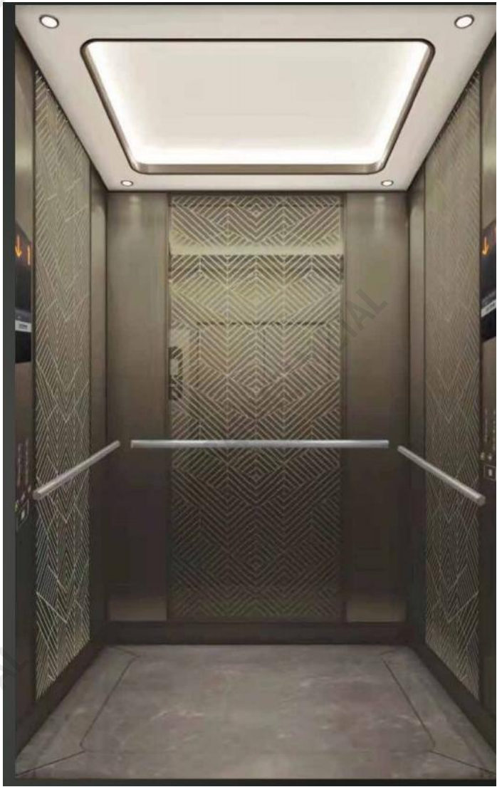
HD121
