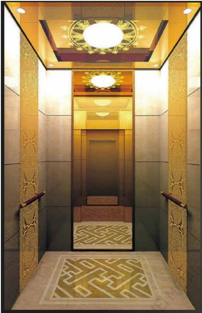
HD 222
