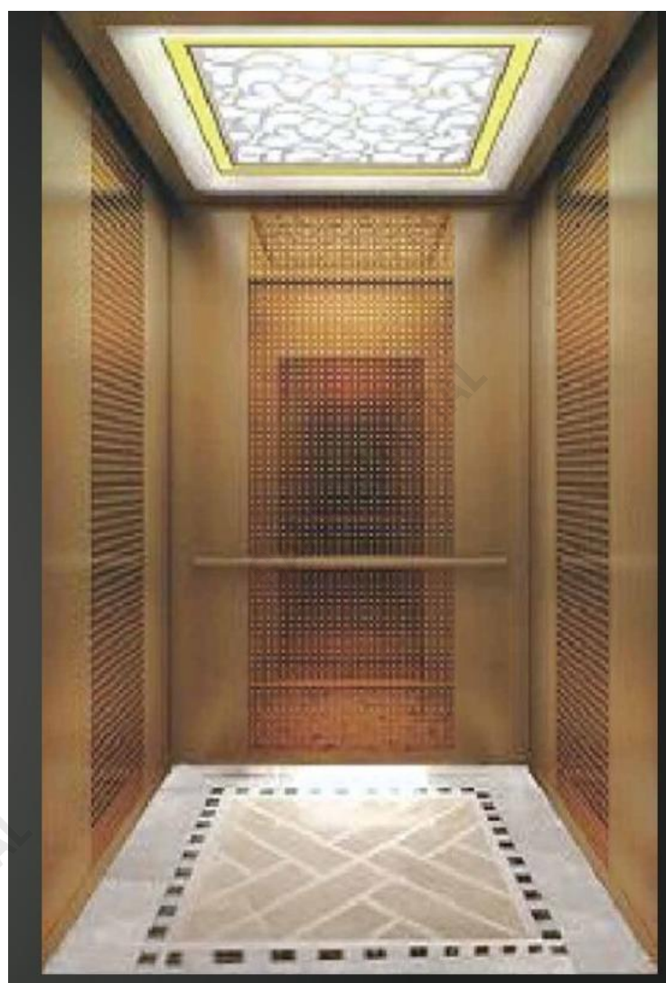
HD212
