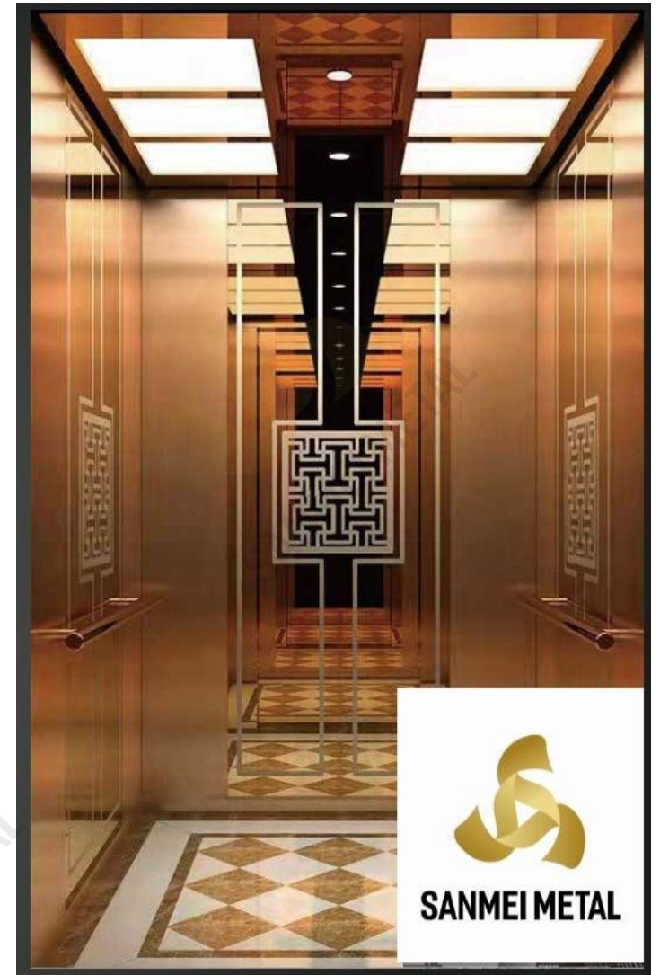
HD218
