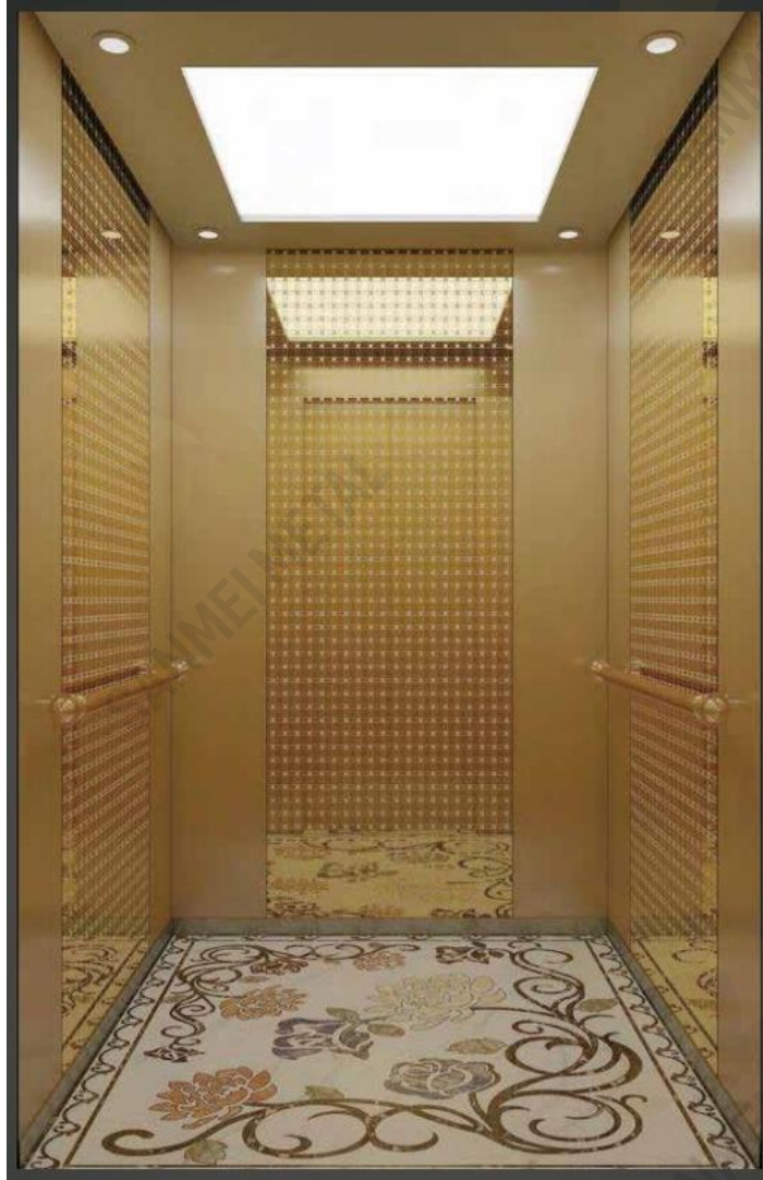
HD 214
