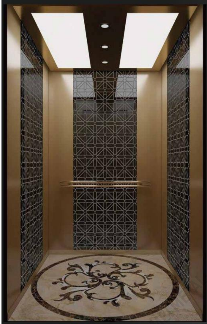
HD 210
