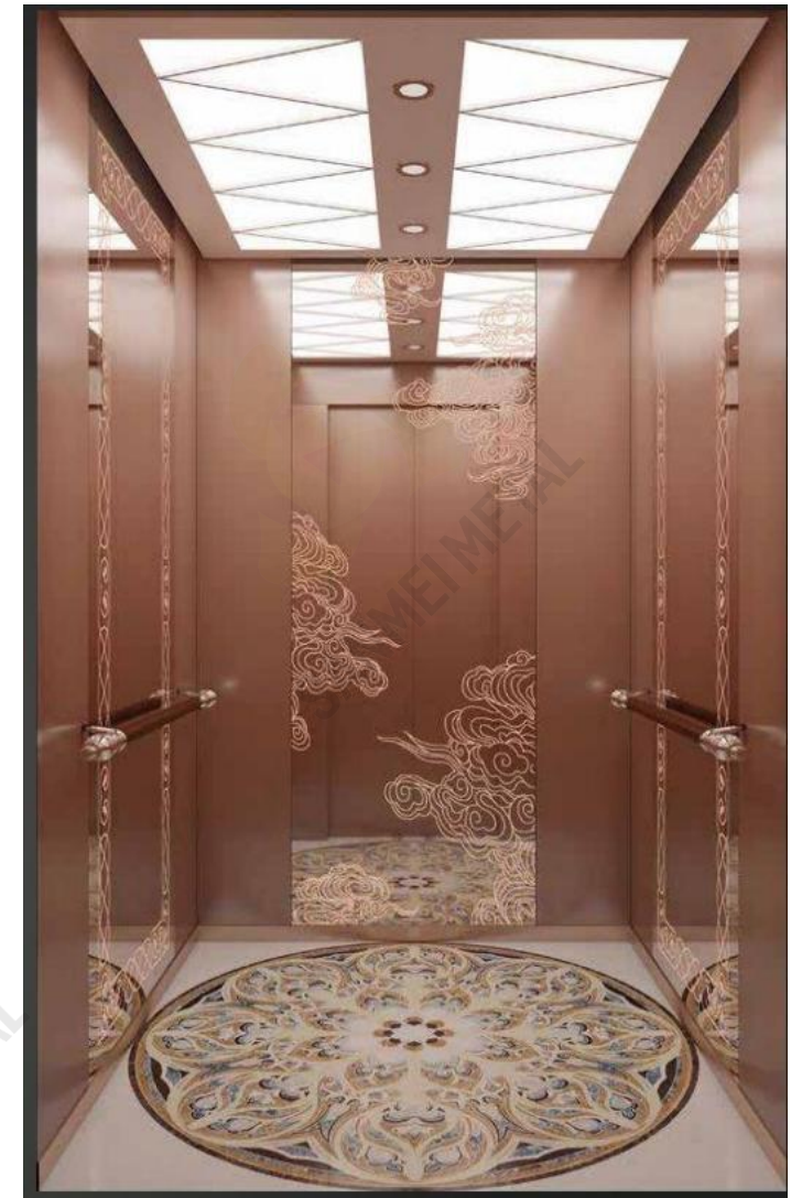
HD206
