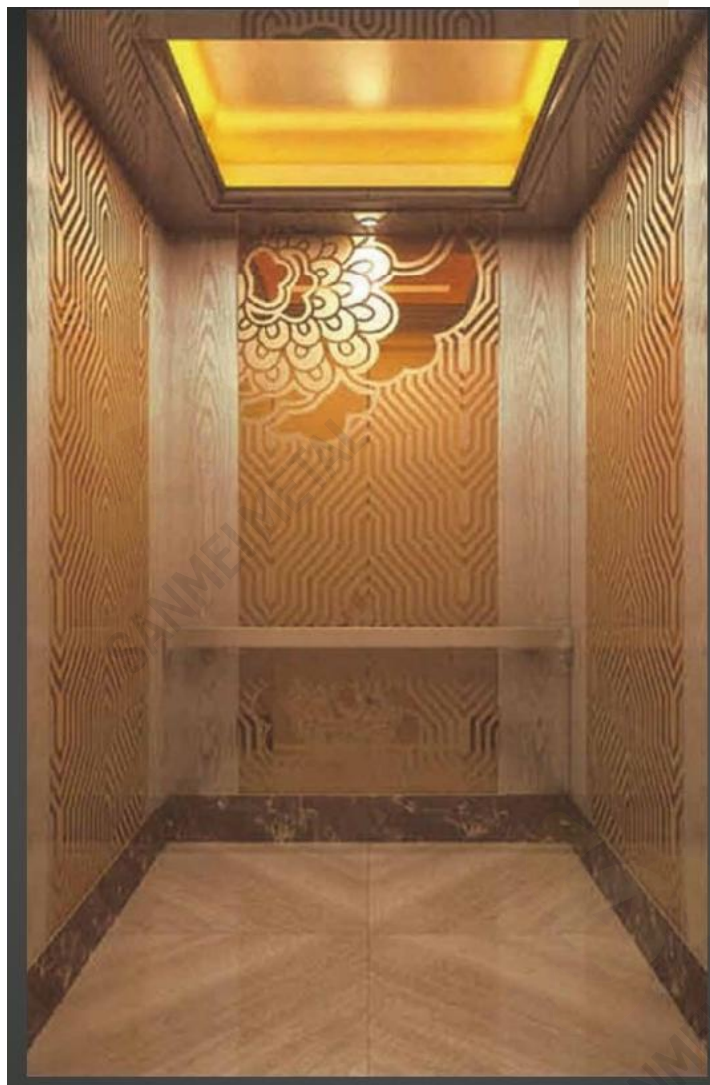
HD 217
